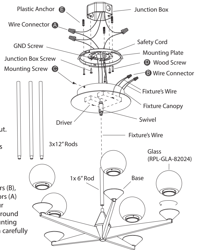
Fig. 2 Wiring
